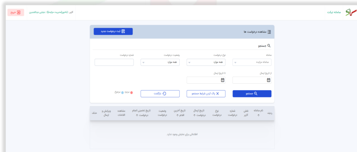
شکل ۳۰- سامانه تیکت
