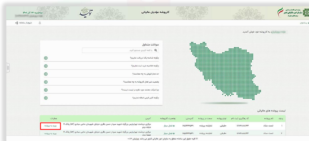
شکل ۶- پنل کاربری
